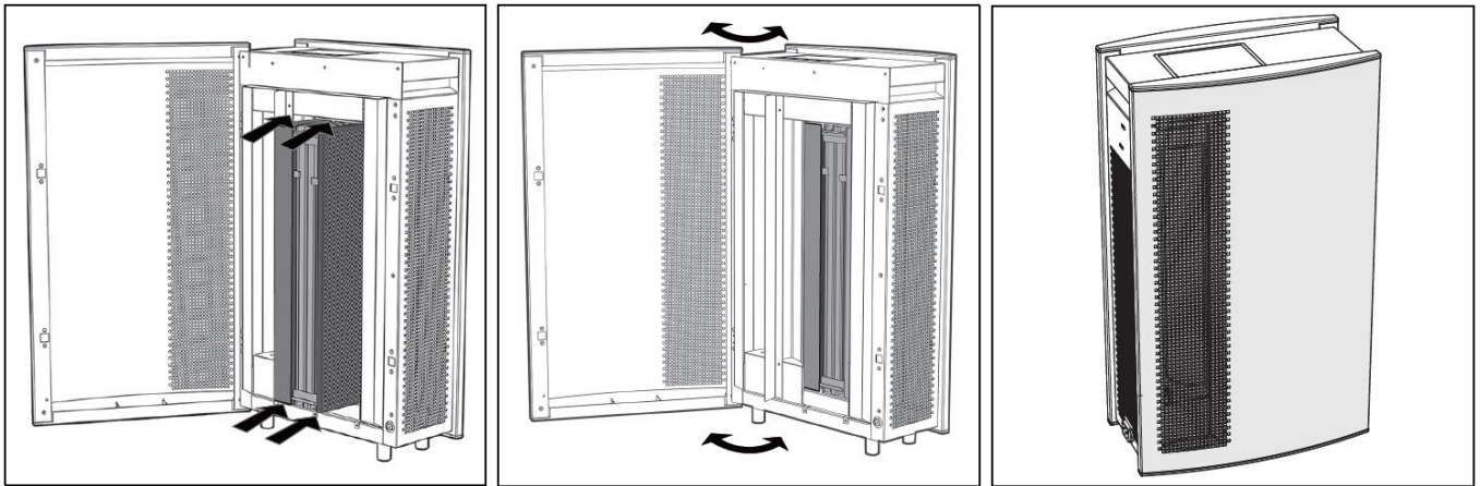
Filtren (schema):
